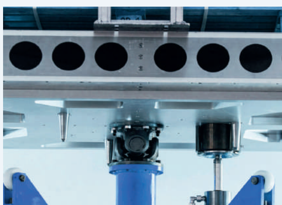
Рис. 9. Пример оснастки
