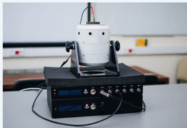
Рис. 8. Небольшой электродинамический вибростенд с подключенным датчиком, контроллер и усилитель
