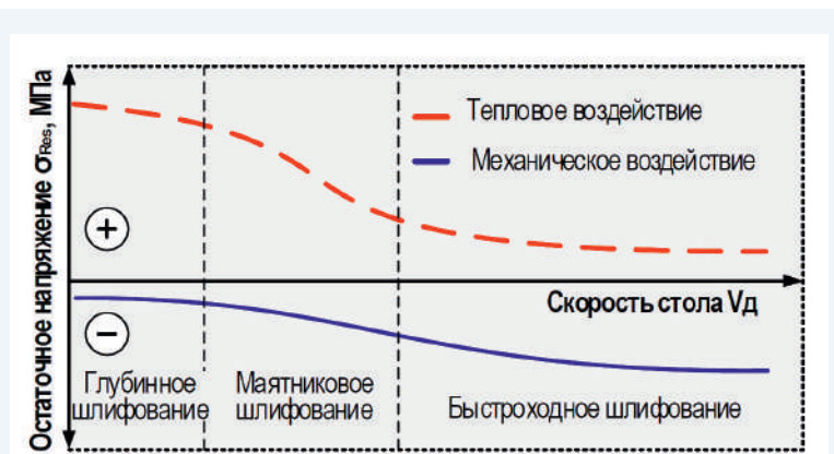
Рис. 6. Изменение остаточных напряжений при скоростном шлифовании закаленной и отпущенной стали шлифовальными кругами из эльбора для разных способов шлифования
