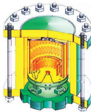
Рис. 1. ГИП шпильной конструкции
