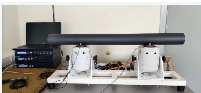
Рис. 4. Использование при испытаниях двух вибростендов
