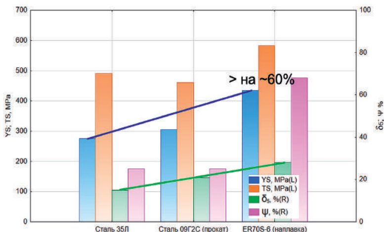
Рис. 2. Механическое совершенствование материалов в технологии WAAM
