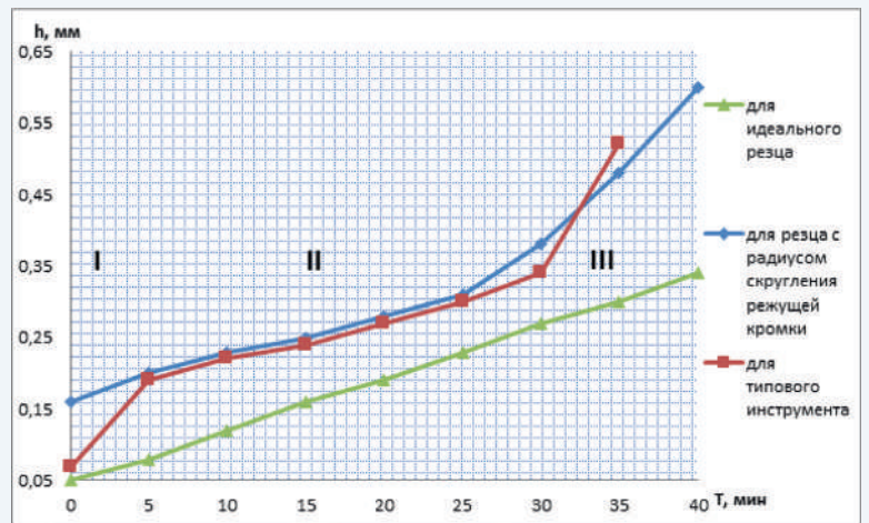
Рис. 2. Зависимость износа от времени работы инструмента. Для типового инструмента: I — зона приработки; II — зона нормальной работы; III — зона катастрофического износа
