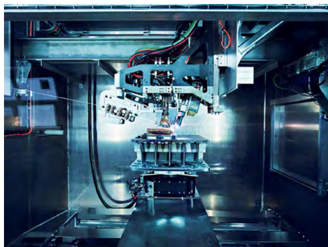
Рис. 6. Система плазменной наплавки с использованием проволоки Norsk Titanium [5]
