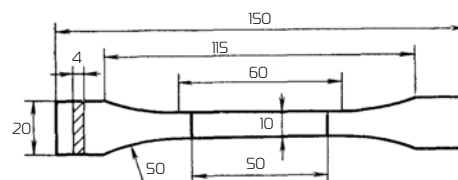
Рис. 1. Эскиз образца для проведения испытаний на растяжение
