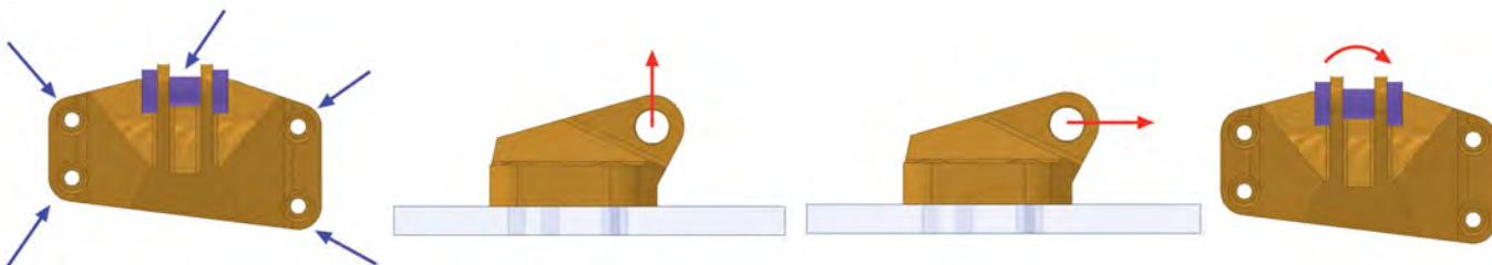
Рис. 4. Определение функций выбранной геометрии
