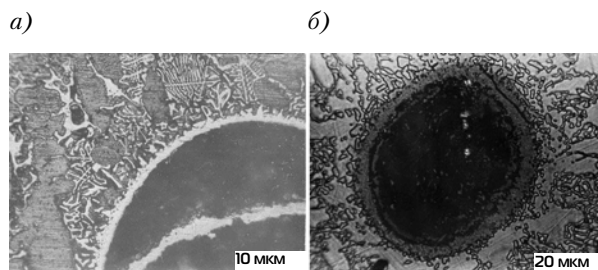
Рис. 7. Микроструктура наплавленного слоя самофлюсующегося никель-хромового сплава ПГ-10 Н-01 с 45% карбидом вольфрама
