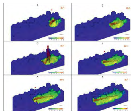
Рис. 2. Вид сбоку на затвердевший слой. Расчет показывает наличие пористости и трещин
