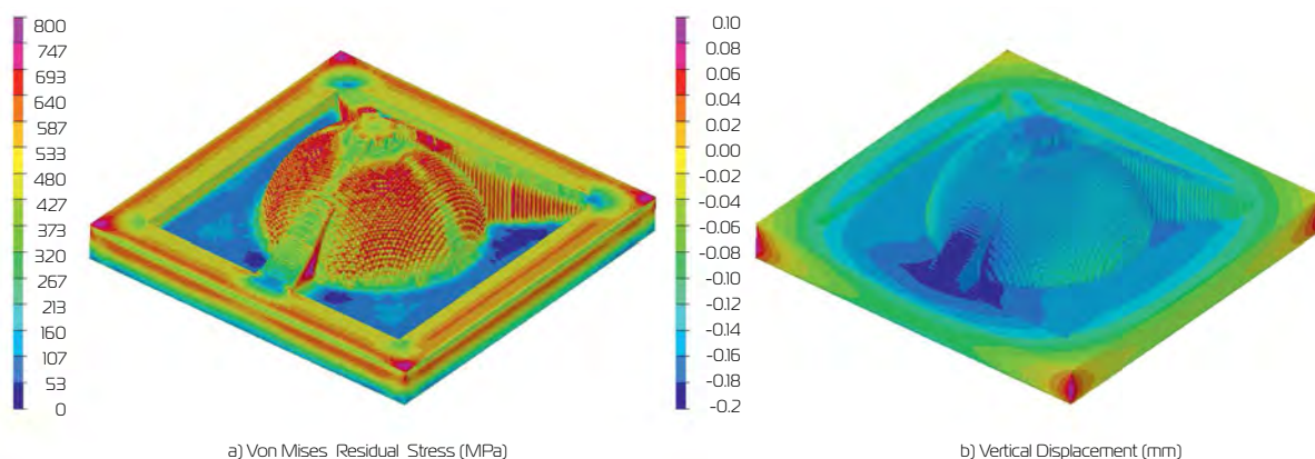
Рис. 3. Распределение напряжений и короблений в заготовке
