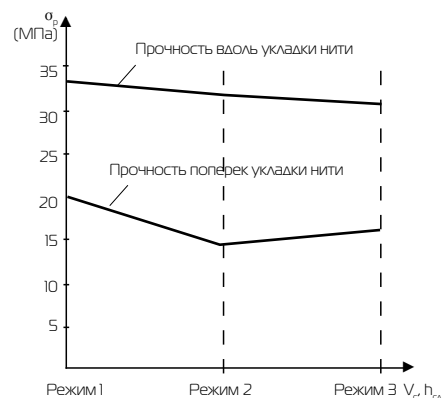
Рис. 2. Зависимость прочности на растяжение \sigma_r модельного материала с продольной и поперечной укладкой нитей, полученного при разных режимах 3D-печати (Режим 1: V_c = 30 мм/сек, h_{cl} = 100 мкм; Режим 2: V_c = 45 мм/сек, h_{cl} = 150 мкм; Режим 3: V_c = 60 мм/сек, h_{cl} = 200 мкм.)
