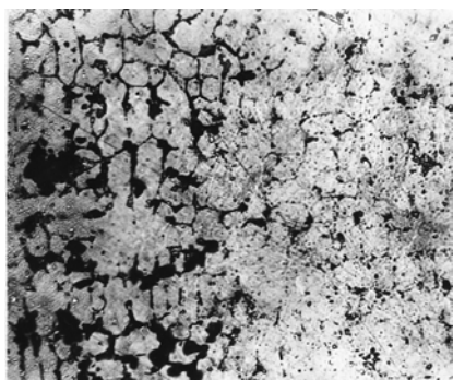
Рис. 5. Микроструктура наплавленной стали Р6М5 во фронте движения лазерного луча и после повторной лазерной переплавки
