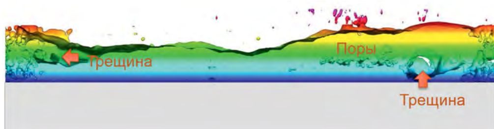
Рис. 2. Вид сбоку на затвердевший слой. Расчет показывает наличие пористости и трещин
