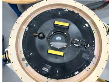
Рис. 1. Пример детали для двери док-станции, отпечатанной на 3D-принтере
