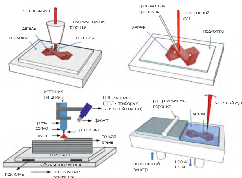
Рис. 1. Схематическое представление АТ (a) DED-L, (b) DED-EB, (c) DED-GMA, (d) PBF-L [1,19]
