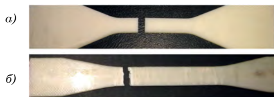
Рис. 3. Характер разрушения образцов с поперечной (а) и продольной (б) укладкой нитей
