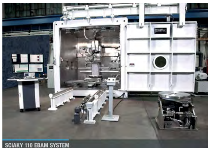
Рис. 5. Система Sciaky EBAM 110 [9, 10]
