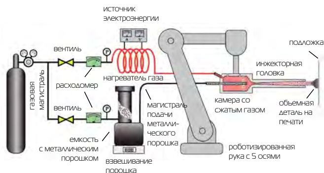
Рис. 2. Схема ХГН-процесса
