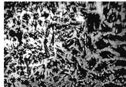
Рис. 4. Металлографический анализ наплавки Р6М5. Типичный мартенсит
