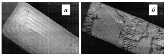
Рис. 4 Вид излома образцов с поперечной (а) и продольной (б) укладкой нитей
