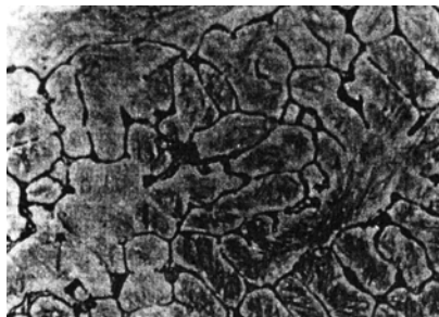
Рис. 3. Металлографический анализ однослойной наплавки стали Р6М5. Распределение карбидов. Масштаб 1:1000
