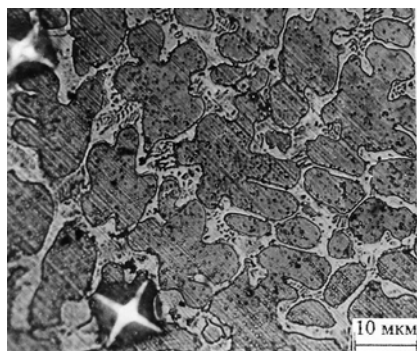
Рис. 2. Микроструктура покрытия ПГ-СРЗ, оплавленного лучом \text{CO}_2 -лазера
