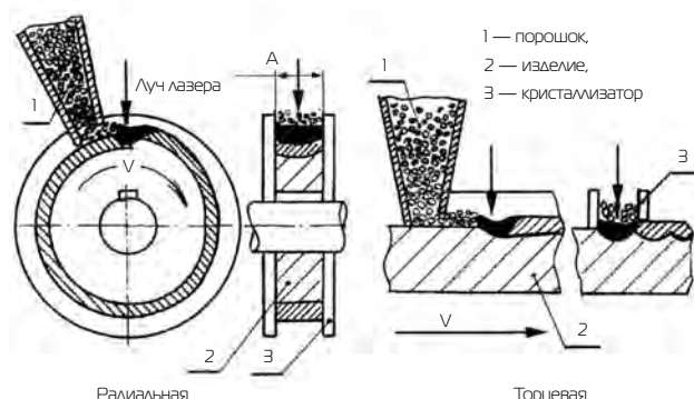
Рис. 1. Схема наплавки
